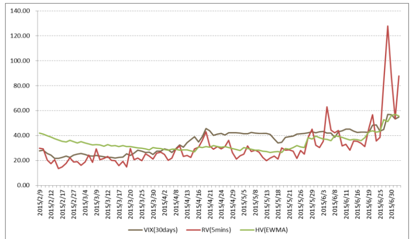
图表 17：50ETF 期权 VIX 指数和标的历史波动率（HV）及已实现波动率（RV）
